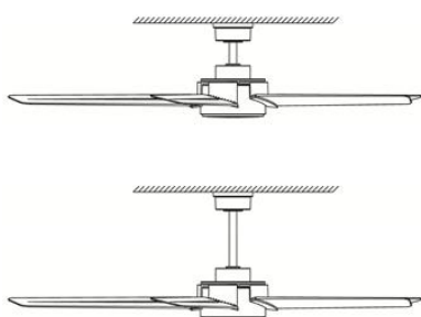
Installation de la tige de suspension
