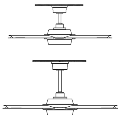
Installation de la tige de suspension
