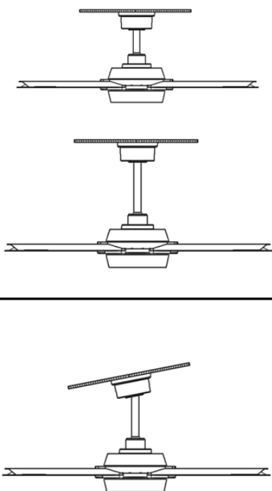
Instalación de varilla
