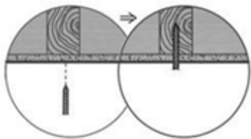
Instalación de tornillo (sin anclaje)
