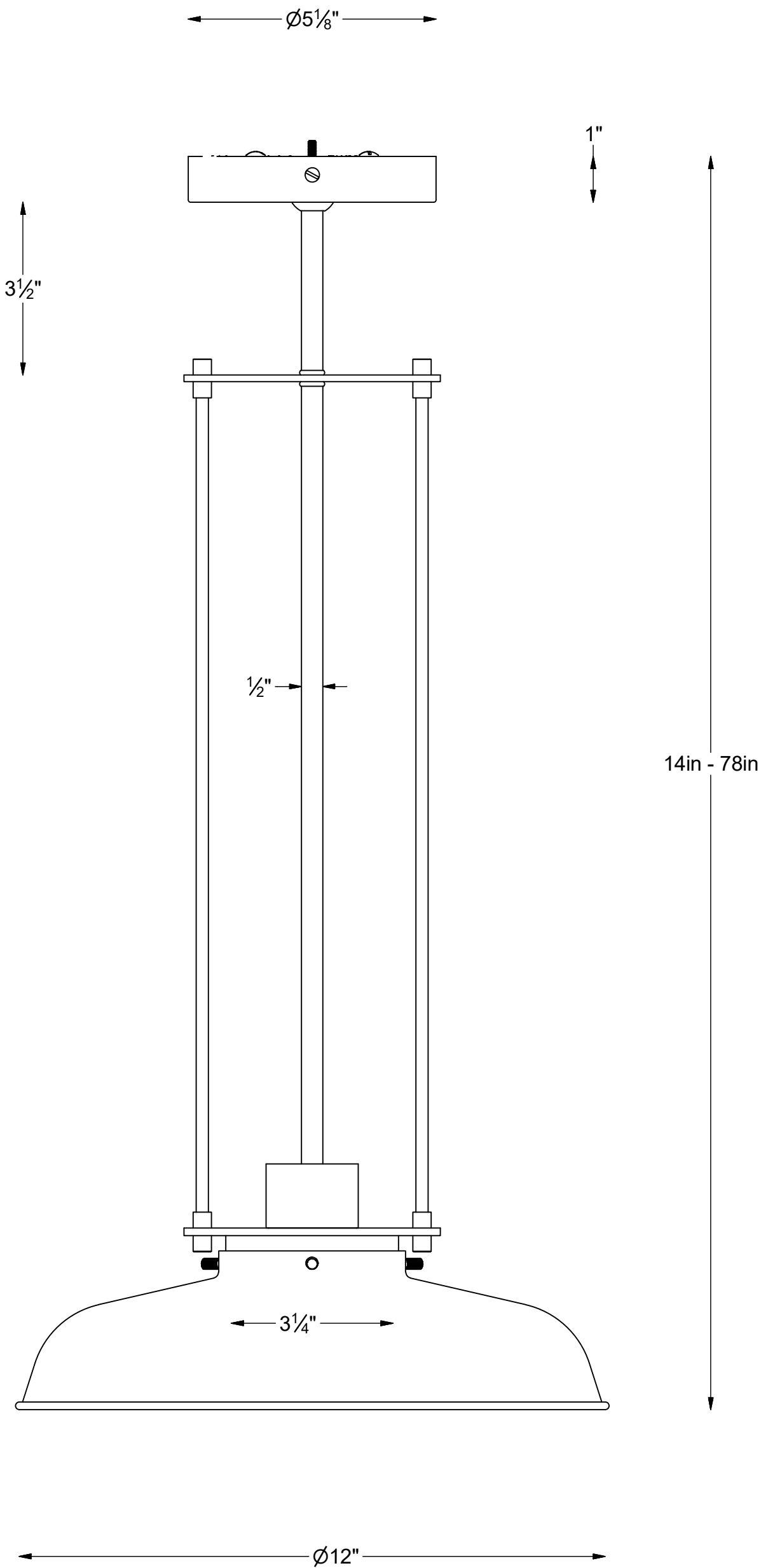
A4335 Ormandy pendant 3-1/4in fitter
