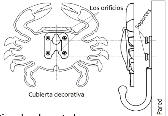
Fig. 3 Presione la cubierta decorativa sobre el soporte de montaje mientras empuja hacia abajo para bloquearla en su lugar.
