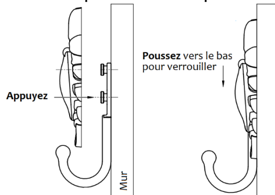
Fig. 3 Appuyez sur le couvercle décoratif sur le support de montage tout en poussant vers le bas pour le verrouiller en place.
