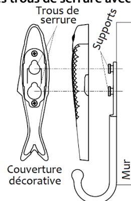
Fig. 3 Appuyez sur le couvercle décoratif sur le support de montage tout en poussant vers le bas pour le verrouiller en place.
