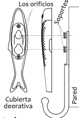
Fig. 3 Presione la cubierta decorativa sobre el soporte de montaje mientras empuja hacia abajo para bloquearla en su lugar.
