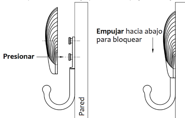
Fig. 3 Presione la cubierta decorativa sobre el soporte de montaje mientras empuja hacia abajo para bloquearla en su lugar.
