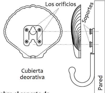
Fig. 3 Presione la cubierta decorativa sobre el soporte de montaje mientras empuja hacia abajo para bloquearla en su lugar.
