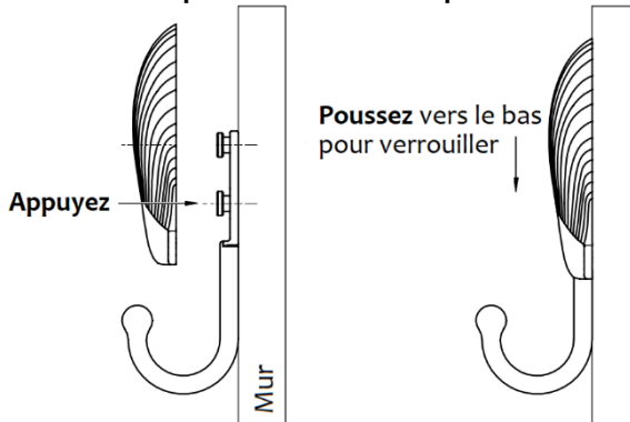
Fig. 3 Appuyez sur le couvercle décoratif sur le support de montage tout en poussant vers le bas pour le verrouiller en place.
