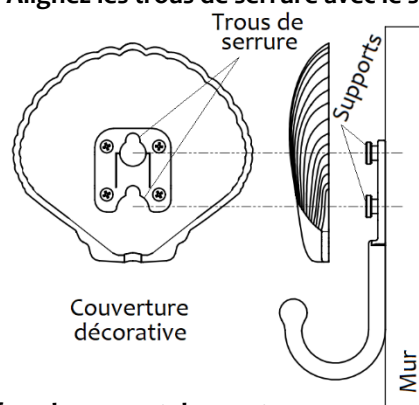
Fig. 3 Appuyez sur le couvercle décoratif sur le support de montage tout en poussant vers le bas pour le verrouiller en place.
