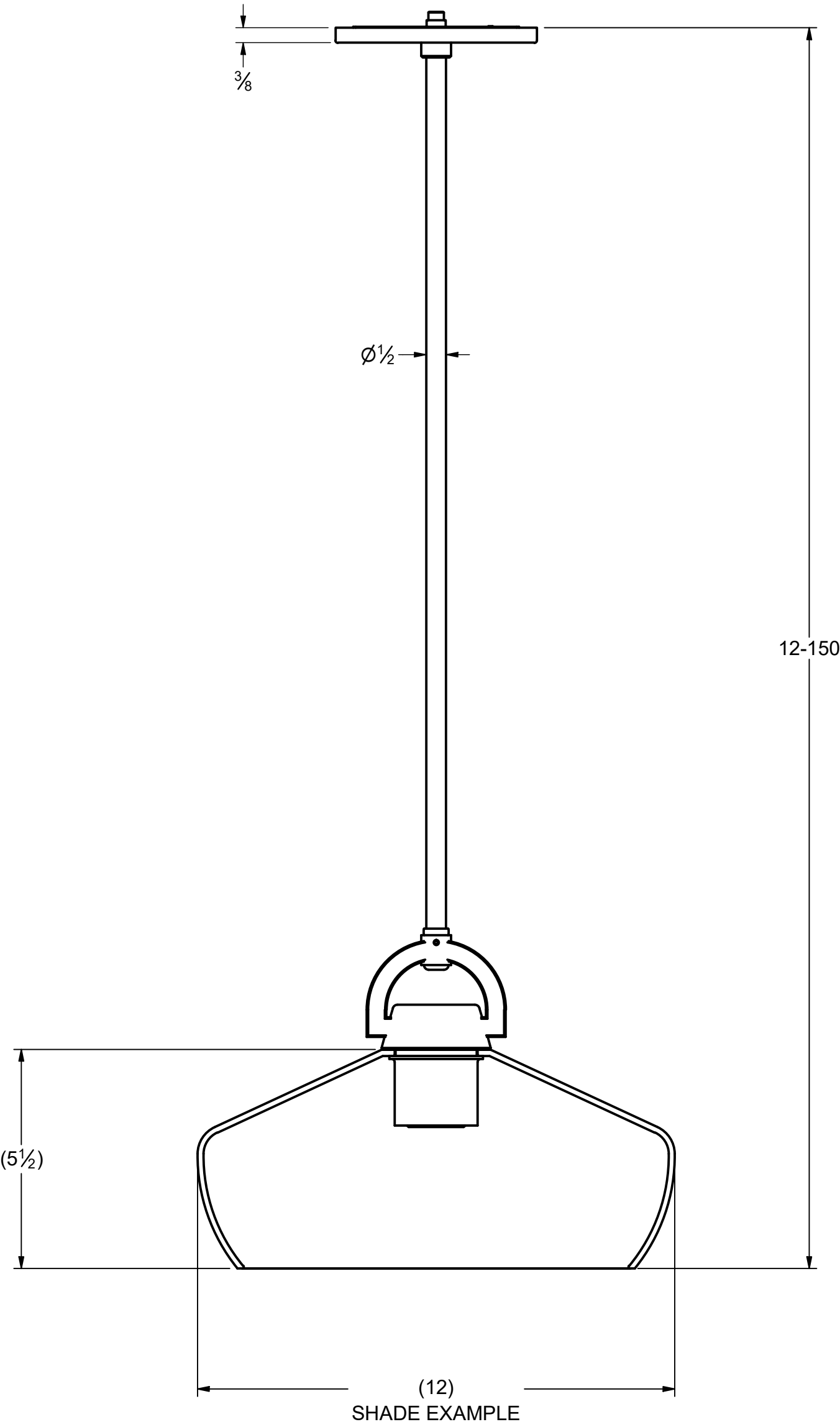
A9358 Whalen Pendant
